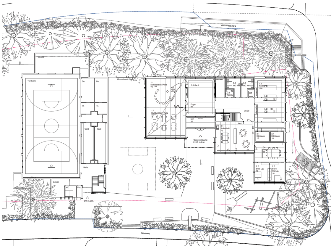
Situation Eingangsgeschoss
